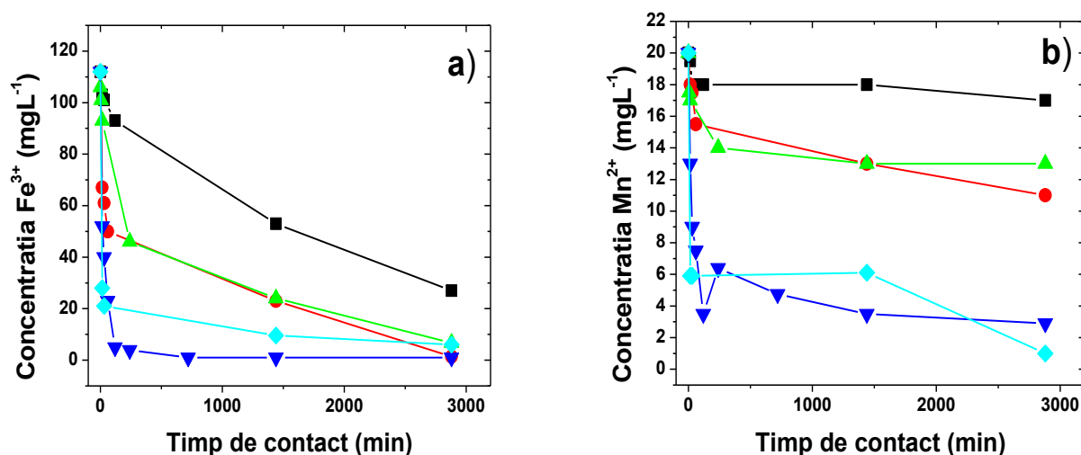
Figura 4. 11. Variația concentrației ionilor de Fe^{3+} (a) și Mn^{2+} (b) din apa acidă de mină în timpul de contact al acestora cu zeolit, în funcție de diferite doze de zeolit (g): (■) 1g, (●) 3g, (▲) 5g, (▼) 10g, (◆) 20g
