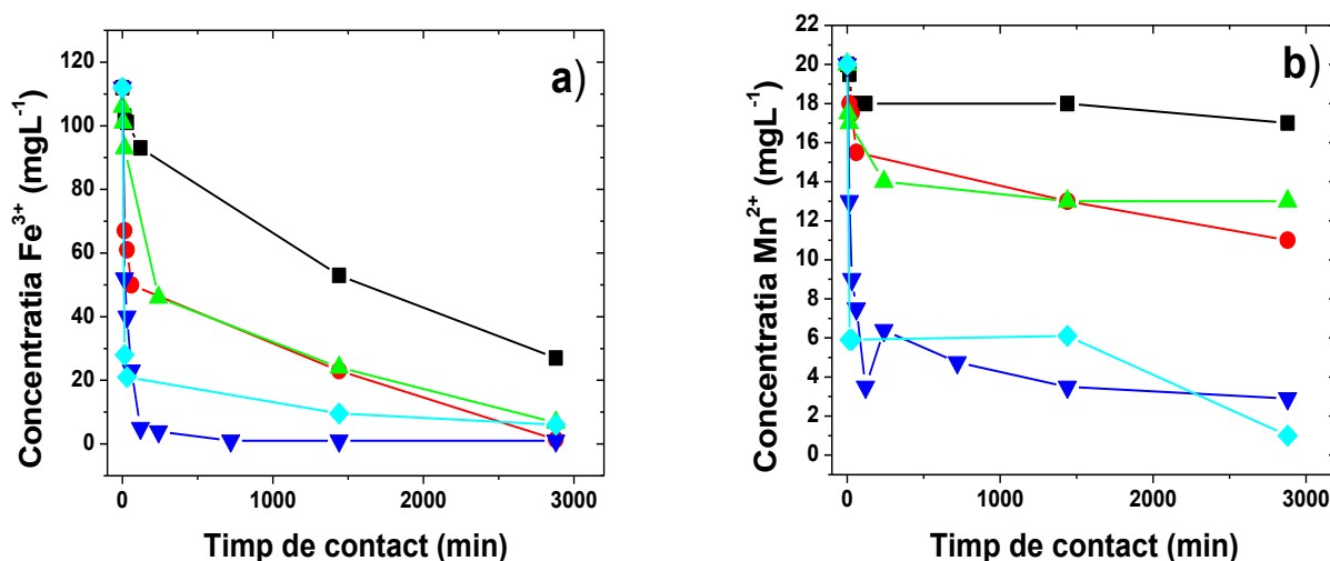
Figura 1.2. Variația concentrației ionilor de Fe^{3+} (a) și Mn^{2+} (b) din apa acidă de mină în timpul de contact al acestora cu zeolit, în funcție de diferite doze de zeolit (g): (■) 1g, (●) 3g, (▲) 5g, (▼) 10g, (◆) 20g
